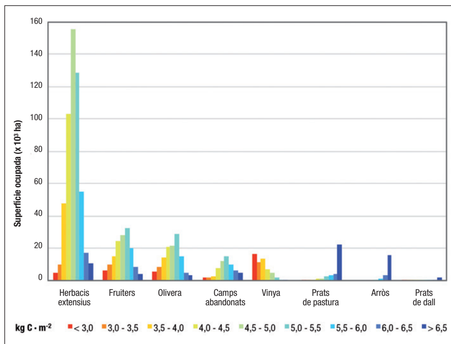
FIGURA 5. Histogrammes de la distribució dels estocs de COS en superfície (kg C·m -2 ) derivada del mapa d'estocs de COS per a cada tipus d'ús de sòl estudiat
