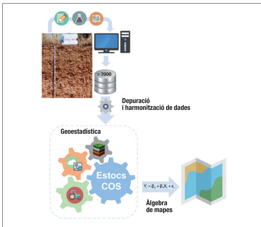
FIGURA 2. Diagrama resum del mètode aplicat per a l'elaboració del mapa dels estocs de COS: obtenció de les dades dels perfils dels sòls, processos de depuració, tractament geoestadístic, algoritmes del mapa resultant
